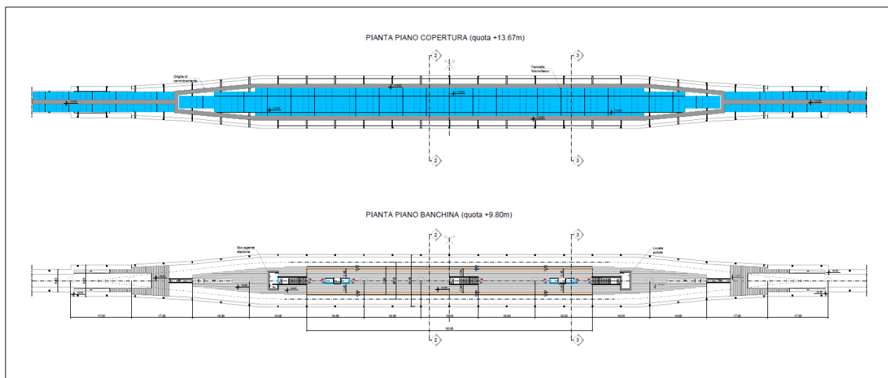
Figura 5. Planimetria tipo delle stazioni
