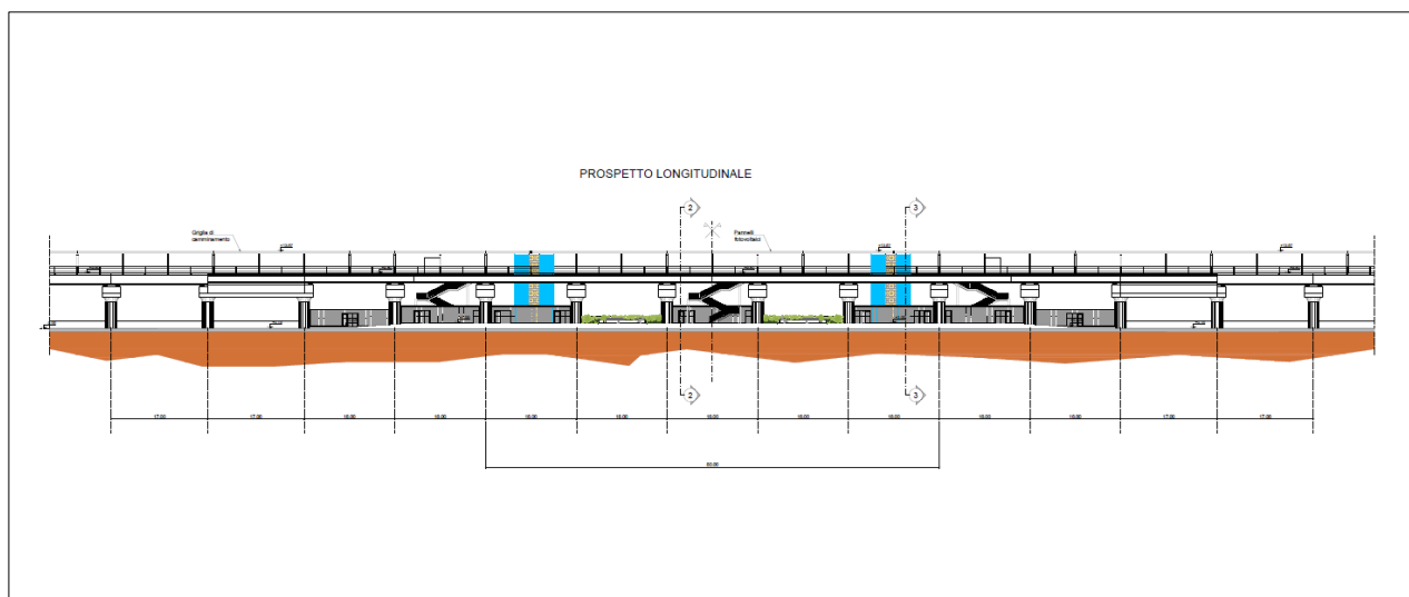
Figura 6. Prospetto longitudinale tipo delle stazioni
