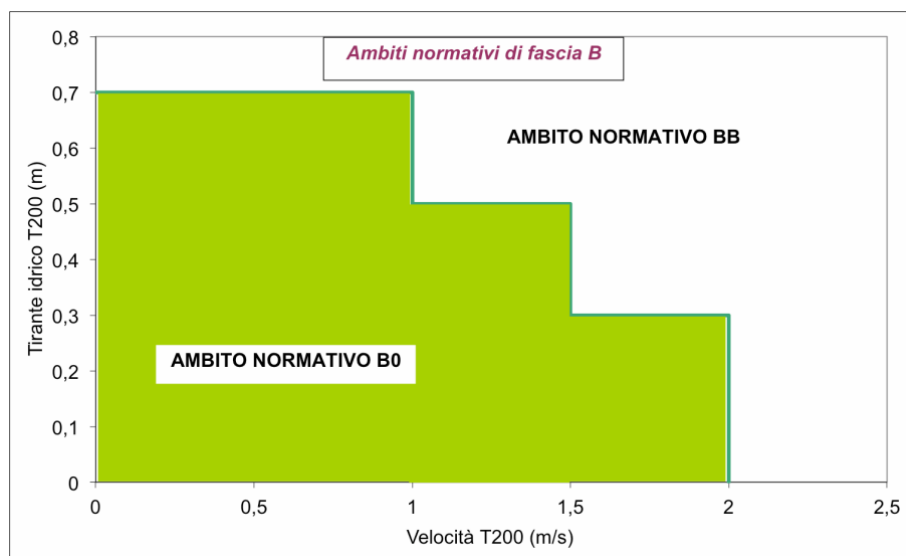
Figura 8. Ambiti normativi di fascia B
