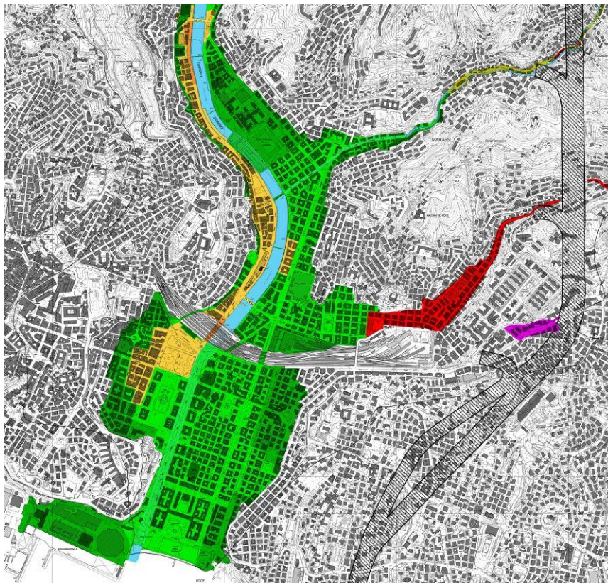
Figura 10. Estratto dalla Carta delle fasce di inondabilità ad efficacia sospesa
