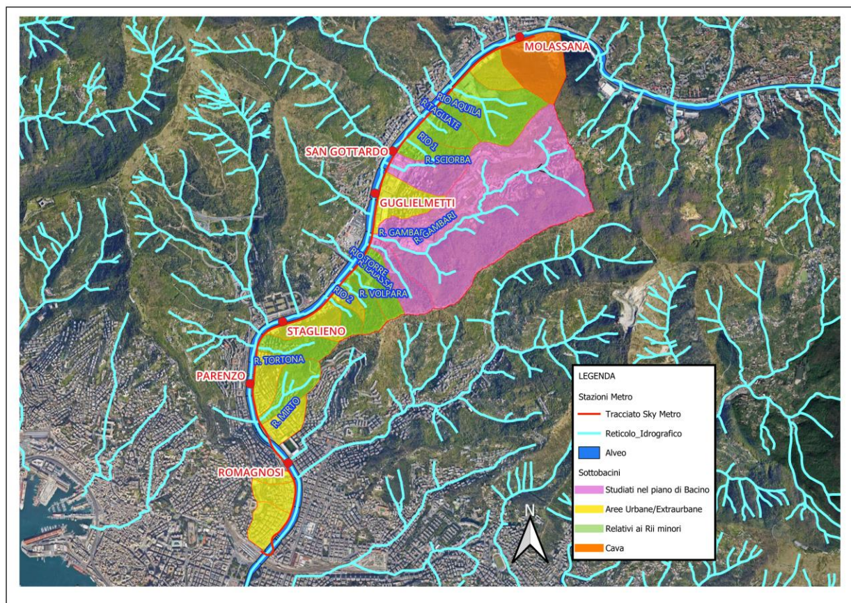
Figura 12. Sottobacini dell'aria di studio
