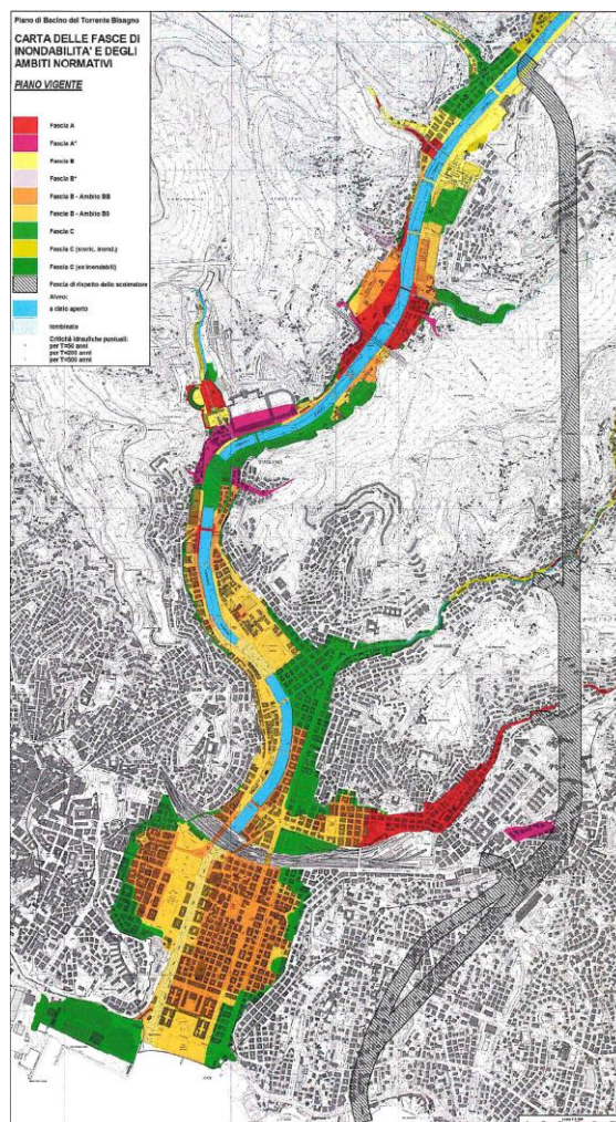
Figura 9. Estratto dalla Carta delle fasce di inondabilità vigente
