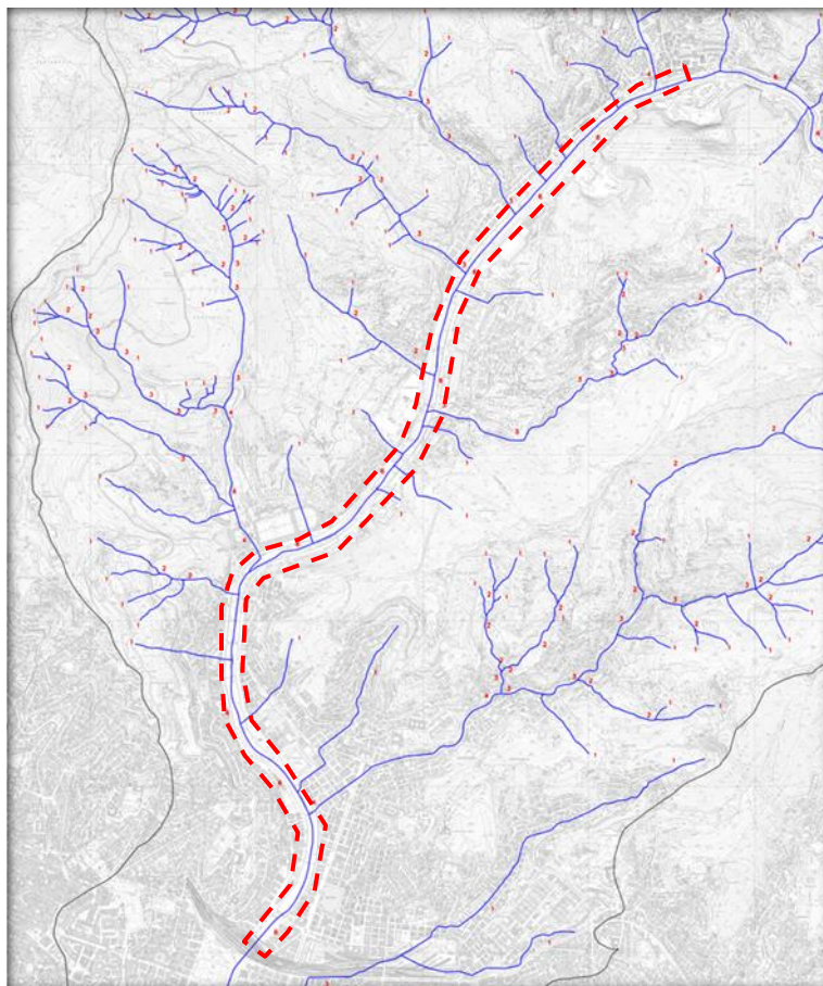
Figura 1. Stralcio cartografico della Carta del reticolo idrografico estratta dal P.d.B. del Torrente Bisagno con ubicazione dell'area in esame
