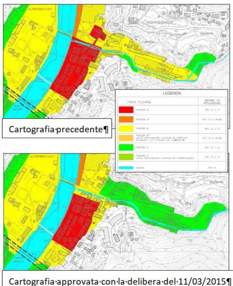
Figura 11. Estratto dalla Carta delle fasce di inondabilità presente nella variante approvata il 11/03/2015 per il rio Mermi
