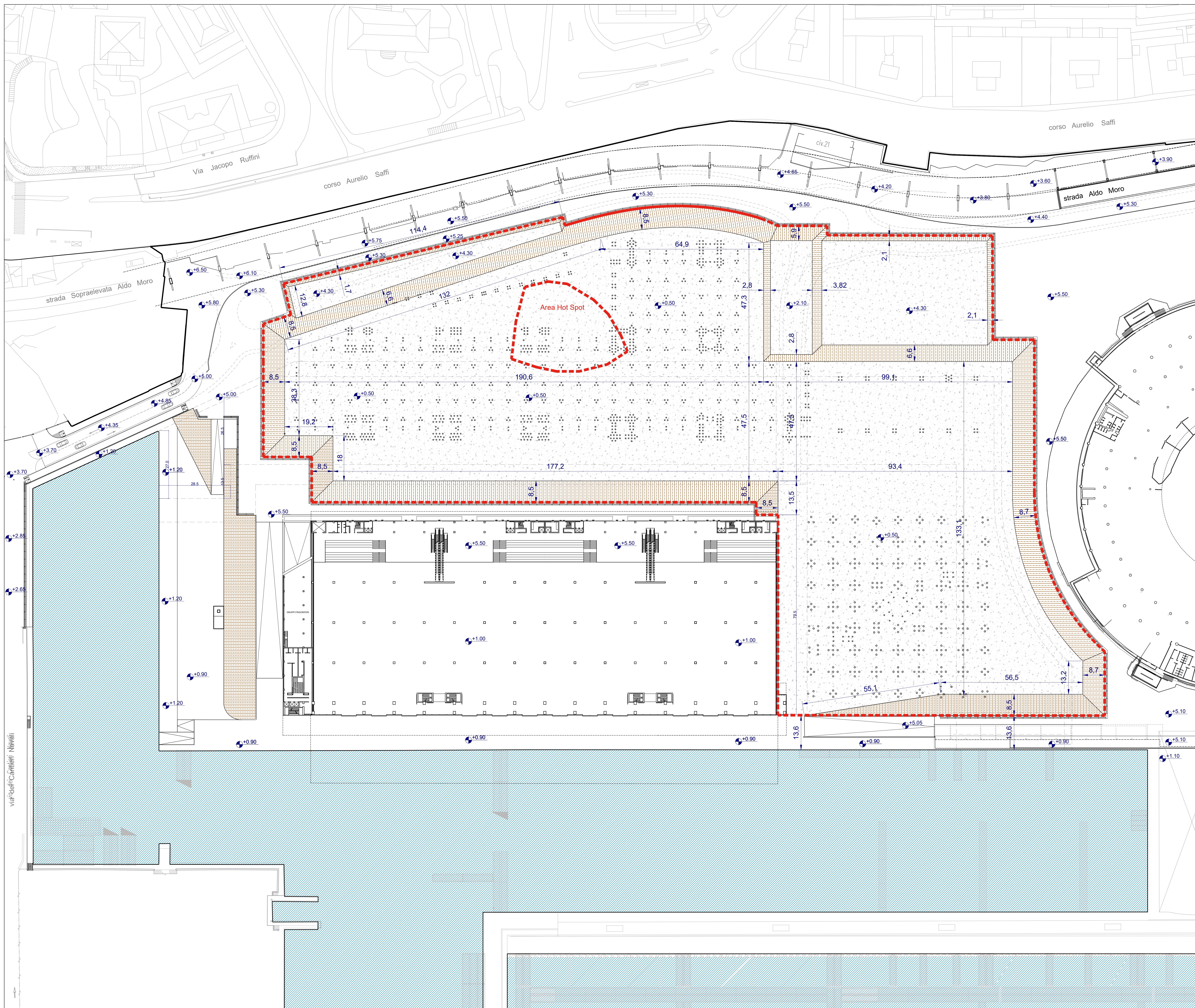
PLANIMETRIA DI PROGETTO - scala 1:500
