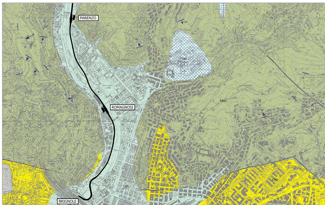
Figura 14. Stralcio carta geomorfologica e geologica inizio intervento Brignole – Parenzo (rif. MGE1PDLGGEOCOMT00100A)
