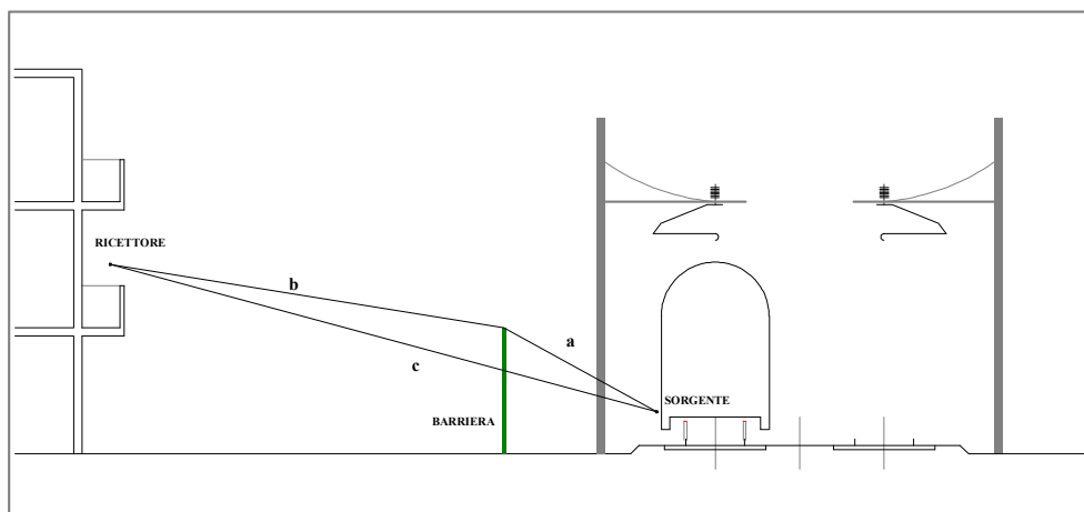
Figura 8. Schematizzazione onde dirette e difratte in presenza di barriere acustiche
