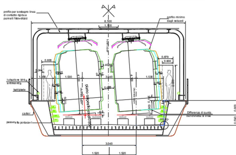
Figura 10. Sezione impalcato a due binari
