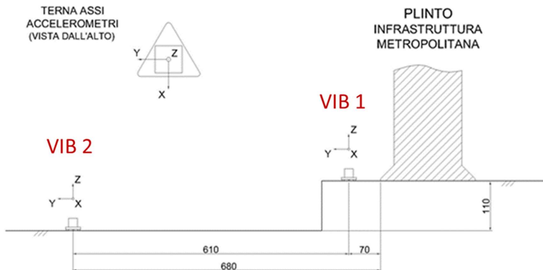
Figura 19. Rilievi in situ: localizzazione dei punti di monitoraggio delle vibrazioni rispetto al piano campagna e piano del ferro
