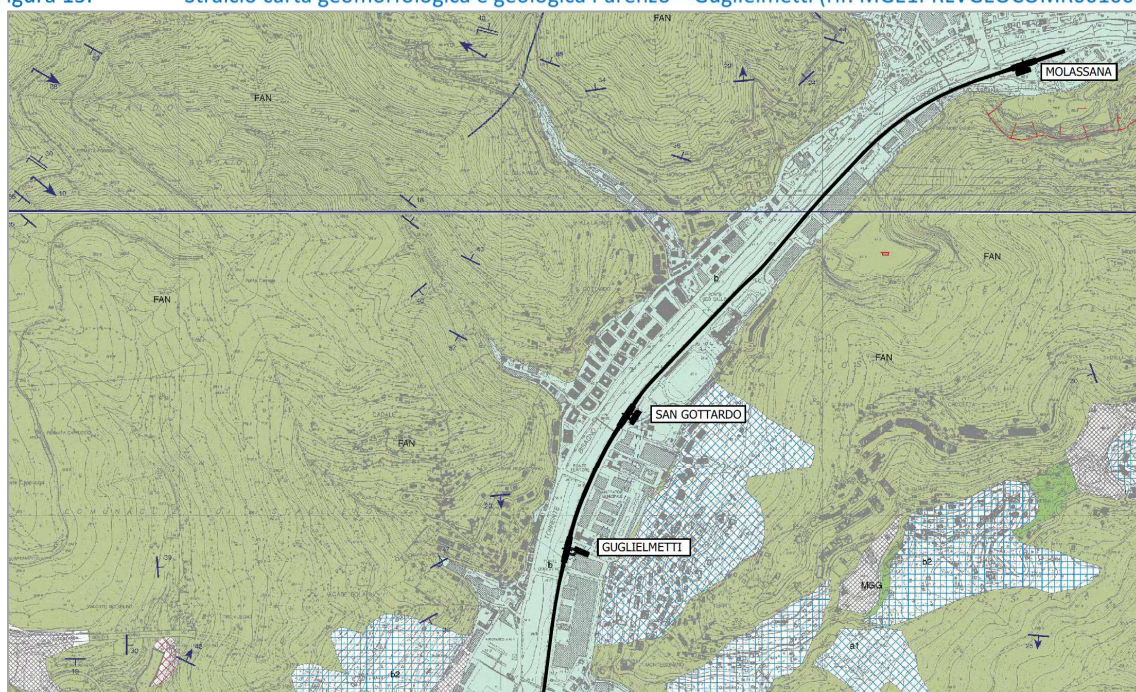
Figura 16. Stralcio carta geomorfologica e geologica fine intervento Guglielmetti – Molassana (rif. MGE1PRLVGEOCOMR00100B)
