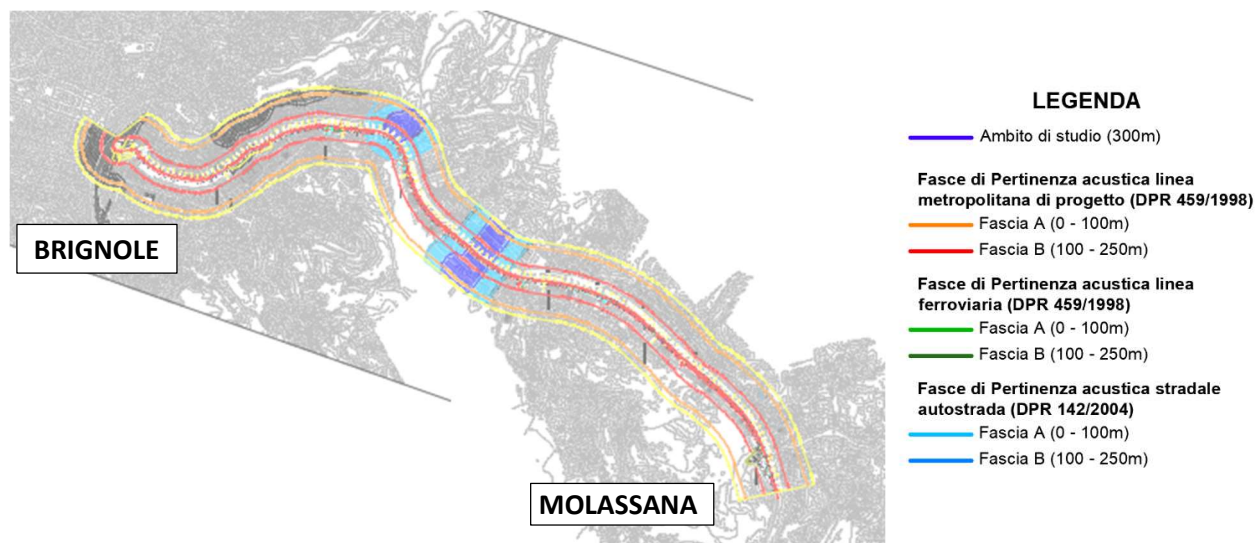
Figura 1. Fasce di pertinenza acustica di progetto
