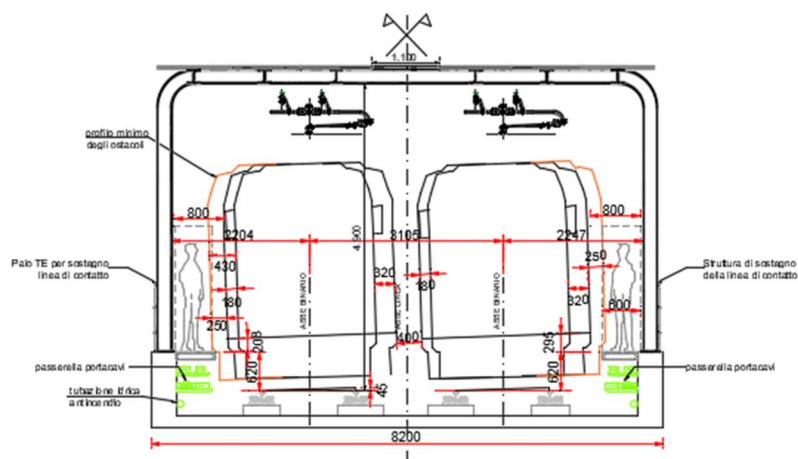
Figura 11. Sezione impalcato Ponte Brignole
