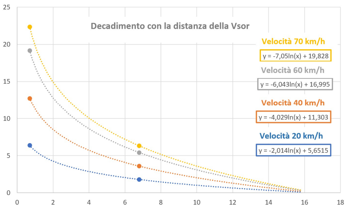
Figura 20. Curve di attenuazione della V sr ricavata dai rilievi nei punti VIB 1 e VIB 2 poste rispettivamente a 0,7 m e 6,8 m dal plinto, ponderate alle velocità di 20 km/h, 40 km/h e 60 km/h
