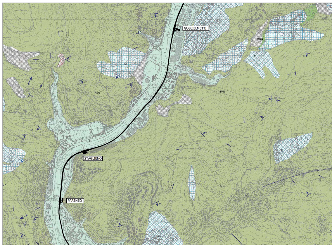
Figura 15. Stralcio carta geomorfologica e geologica Parenzo – Guglielmetti (rif. MGE1PRLVGEOCOMR00100B)
