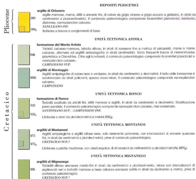
Figura 17. Legenda carta geomorfologica e geologica (rif. MGE1PRLVGEOCOMR00100B)
