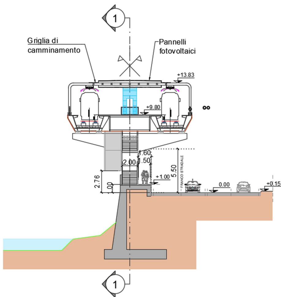
Figura 9. Sezione impalcato in corrispondenza dei marciapiedi di stazione
