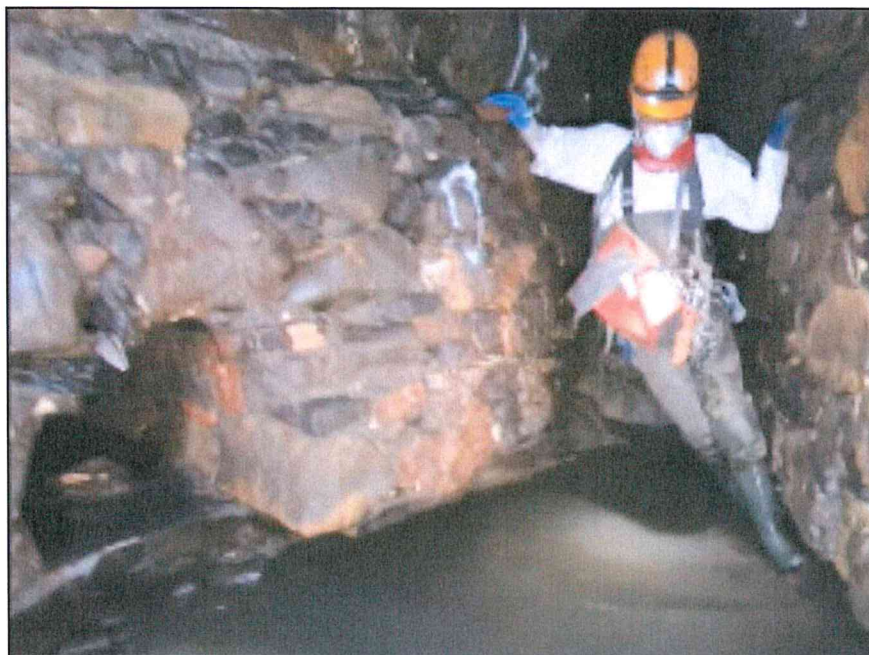
Foto 3 – parziale sgrottamento in corrispondenza delle fondazioni dell'edificio civ. 11 di Corso Dogali
