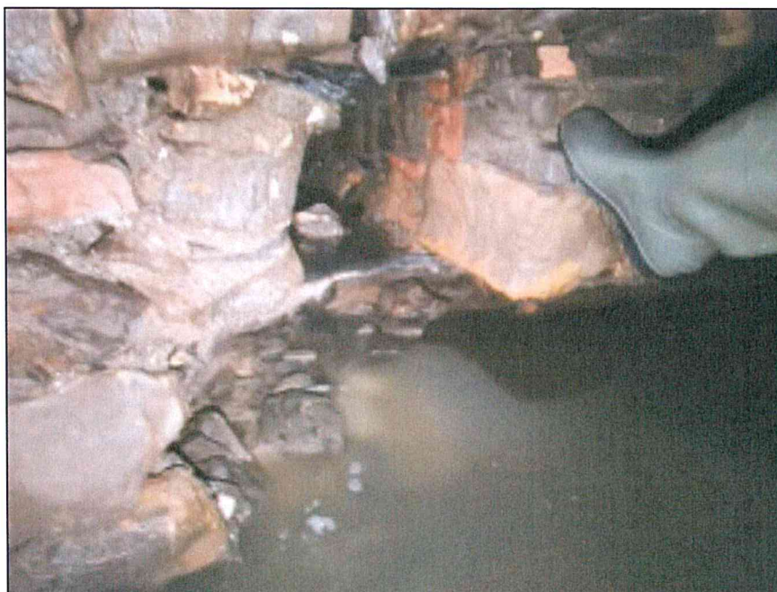
Foto 4 – particolare parziale sgrottamento in corrispondenza delle fondazioni dell'edificio civ. 11 di Corso Dogali
