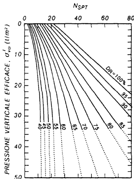
Figura 6-3 – Correlazione di Gibbs ed Holtz (1957)
