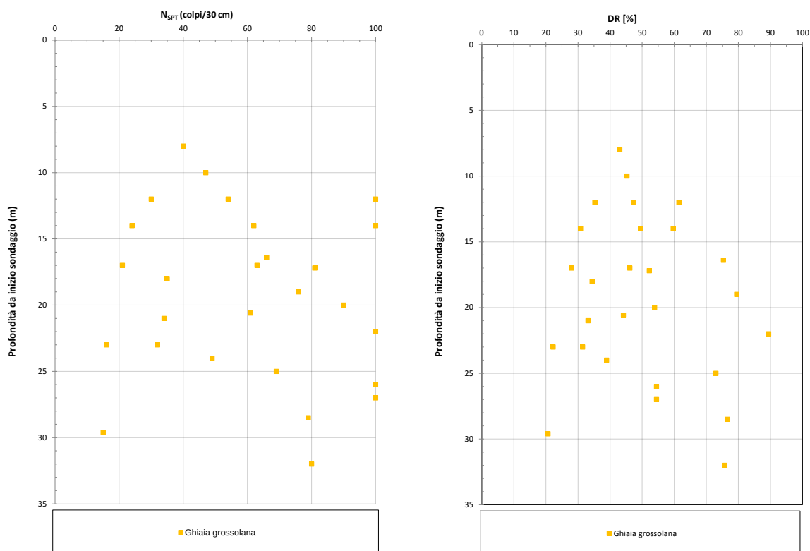
Figura 7-11 – Valori di N_{SPT} a (sx) e densità relativa DR (dx) per l'Unità C (ghiaia grossolana)
