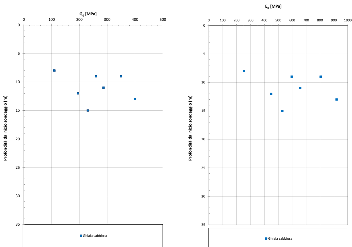
Figura 7-9 – Modulo di taglio G_0 (sx) e Modulo di Young alle piccole deformazioni ( E_0 ) (dx) – Unità B
