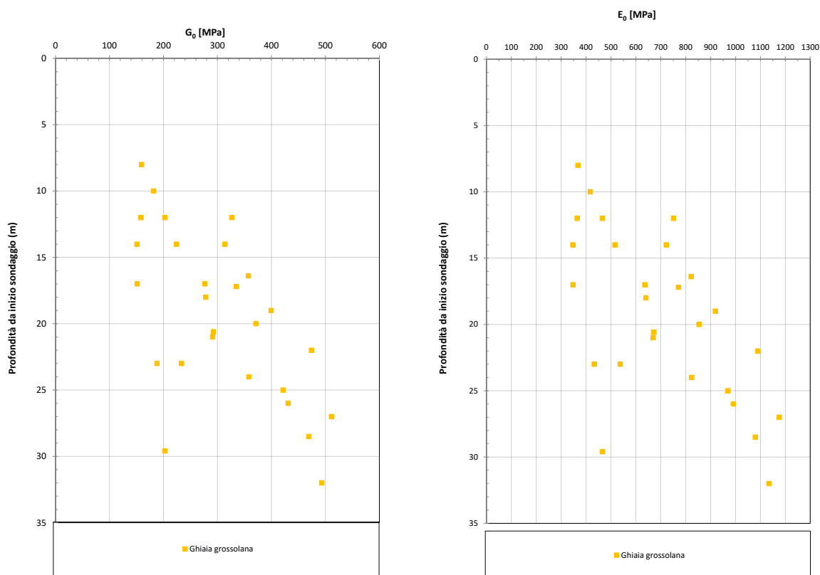
Figura 7-15 – Modulo di taglio G_0 (sx) e Modulo di Young alle piccole deformazioni ( E_0 ) (dx) – Unità C
