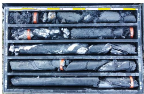
MIF7 (da 25 a 27 m da p.c)
