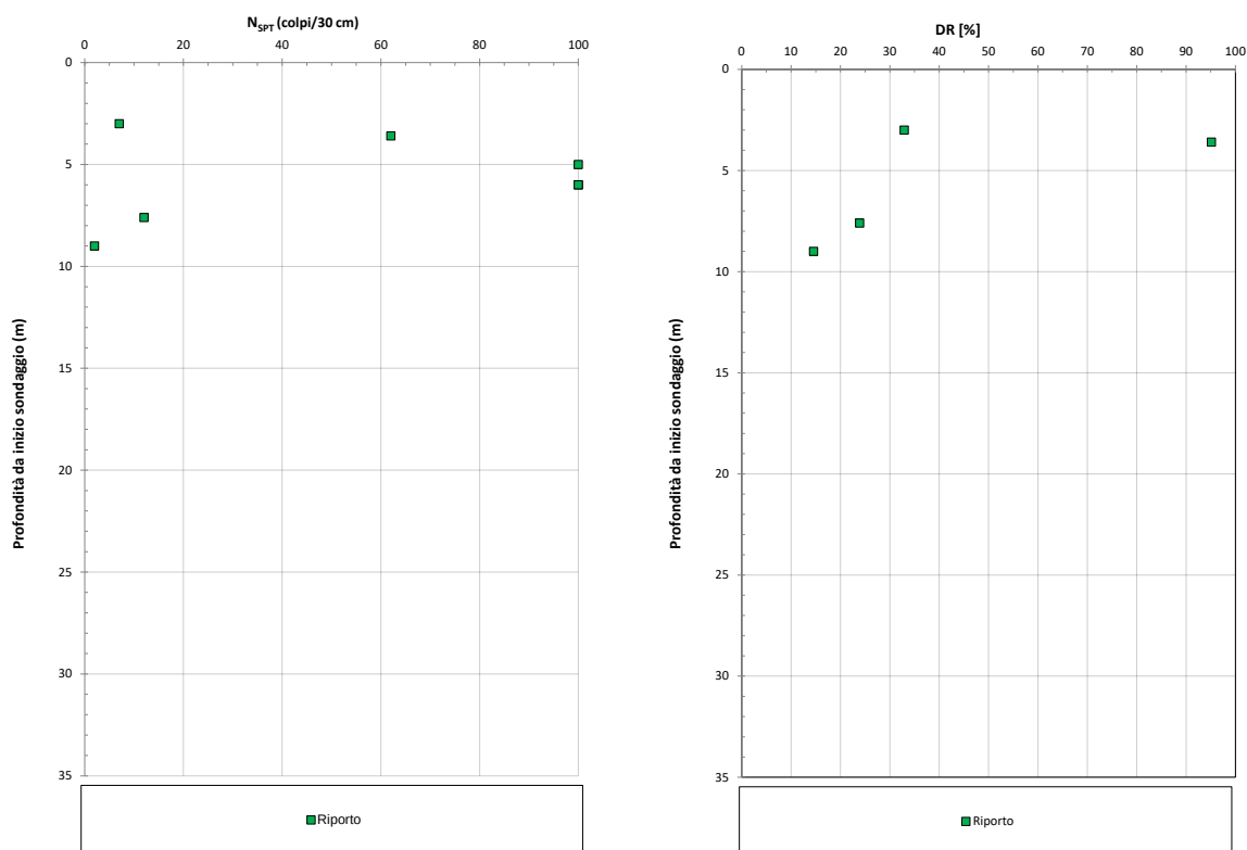
Figura 7-3 – Valori di N_{SPT} a (sx) e densità relativa DR (dx) per l'unità A (Riporto)
