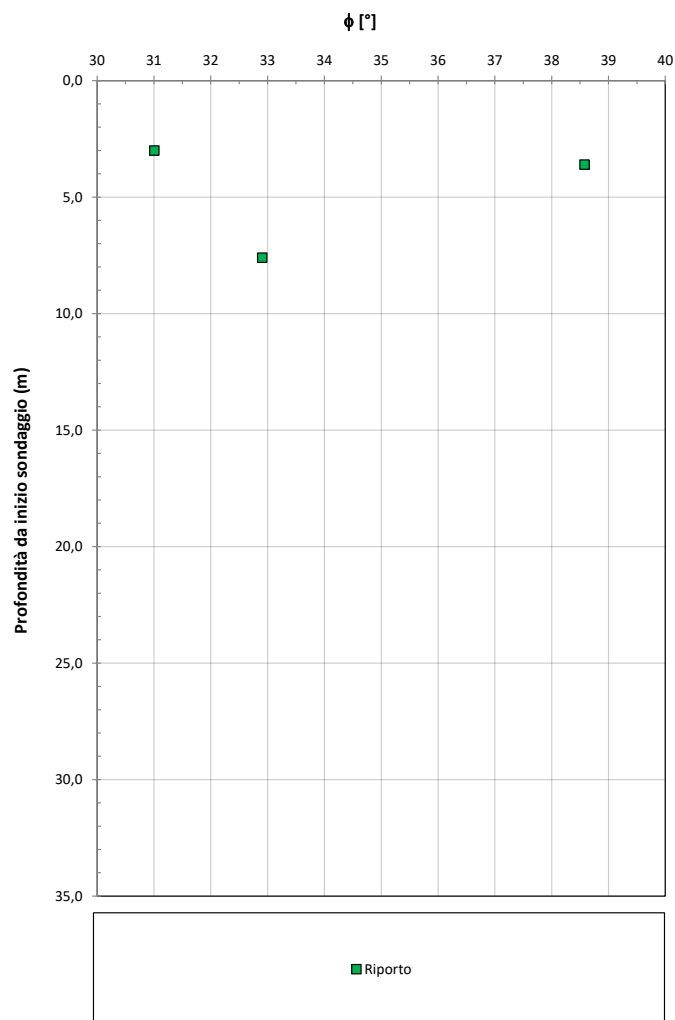
Figura 7-4 – Valori dell'angolo di resistenza al taglio ricavati dalle prove N_{SPT} - Unità A
