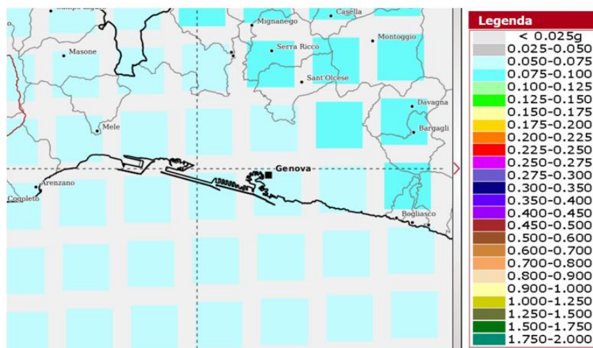
Figura 5-4 – Mappa interattiva di pericolosità sismica (INGV)
