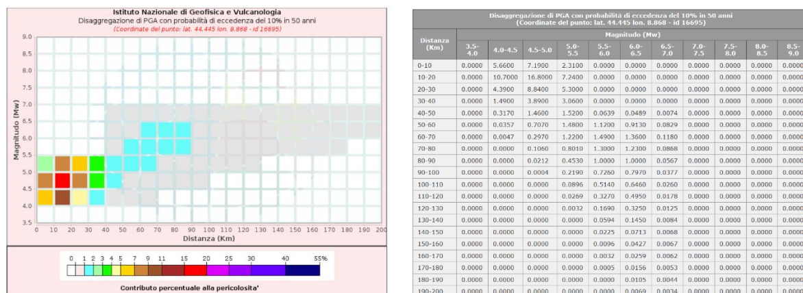
Figura 5-5 - Analisi di disaggregazione per definizione terremoto dominante dell'area
