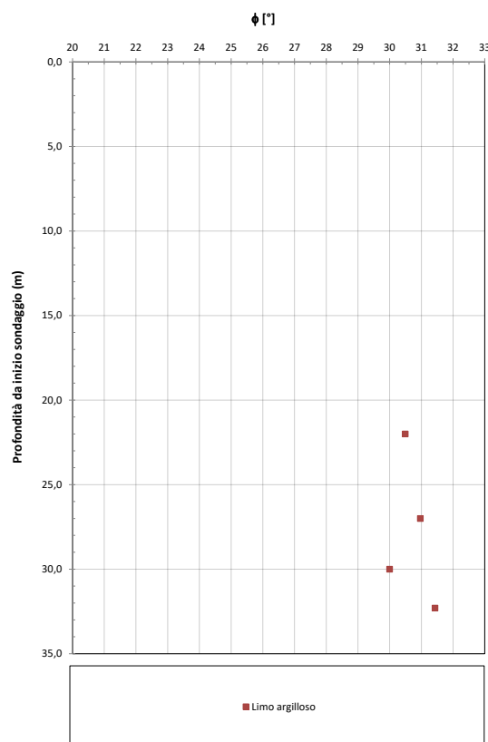
Figura 7-19 – Valori dell'angolo di resistenza al taglio ricavati dalle prove N_{SPT} – Unità D
