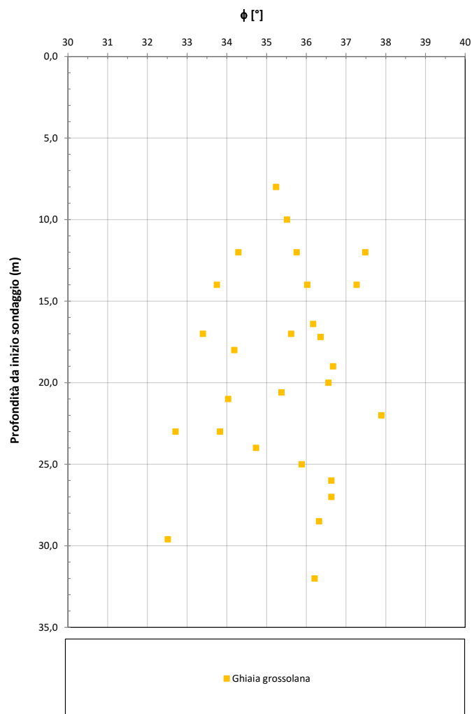
Figura 7-14 – Valori dell'angolo di resistenza al taglio ricavati dalle prove N_{SPT} – Unità C
