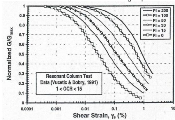
Figura 6-4 – Curve sperimentali del rapporto G/G_{max} da prove di colonna risonante ciclica (Vucetic & Dobry, 1991).
