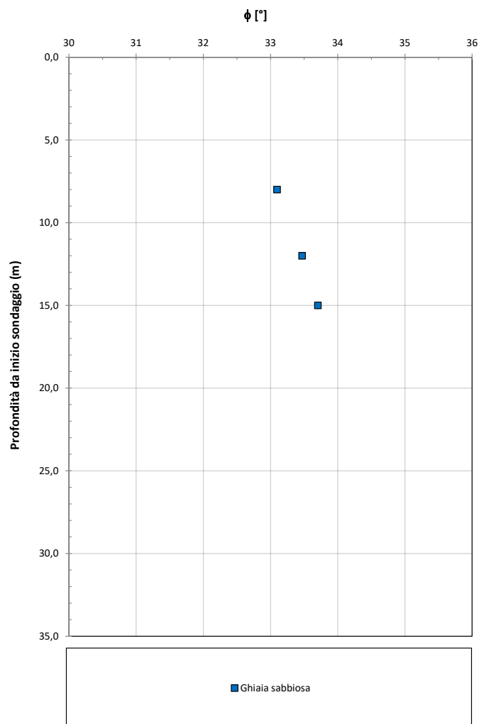
Figura 7-8 – Valori dell'angolo di resistenza al taglio ricavati dalle prove N_{SPT} – Unità B
