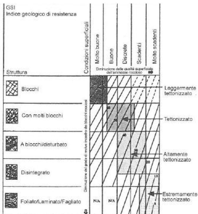
Figura 6-5 - Carta del GSI (Hoek et al., 1998)
