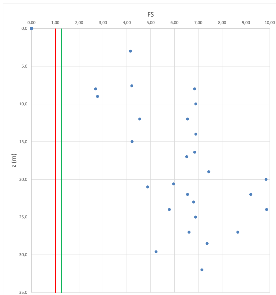
Figura 5-7 – Fs da verifica di liquefazione
