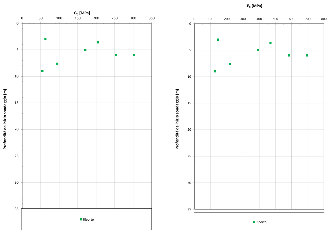
Figura 7-5 – Modulo di taglio G_0 (sx) e Modulo di Young alle piccole deformazioni ( E_0 ) (dx) - Unità A
