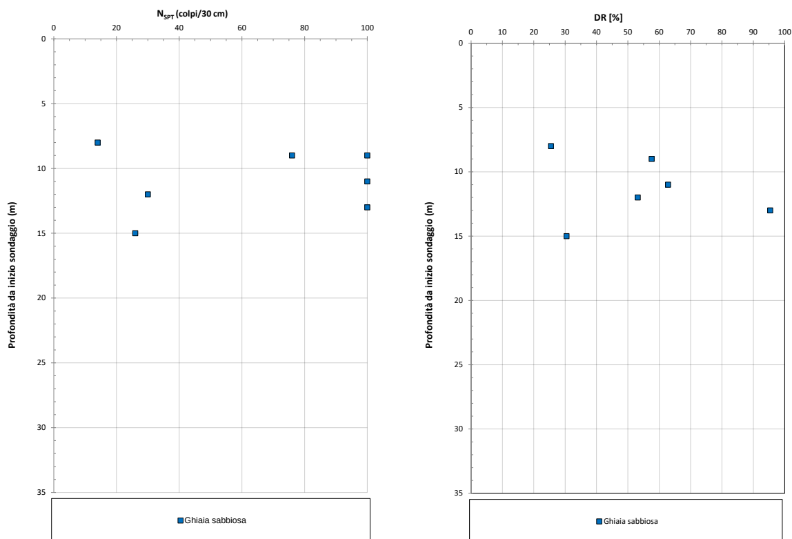
Figura 7-7 – Valori di N_{SPT} (sx) e densità relativa DR (dx) per l'unità B (Ghiaia sabbiosa limosa)
