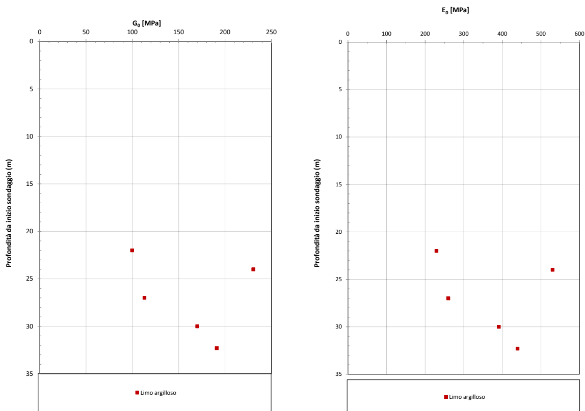
Figura 7-20 – Modulo di taglio G_0 (sx) e Modulo di Young alle piccole deformazioni ( E_0 ) (dx) – Unità D
