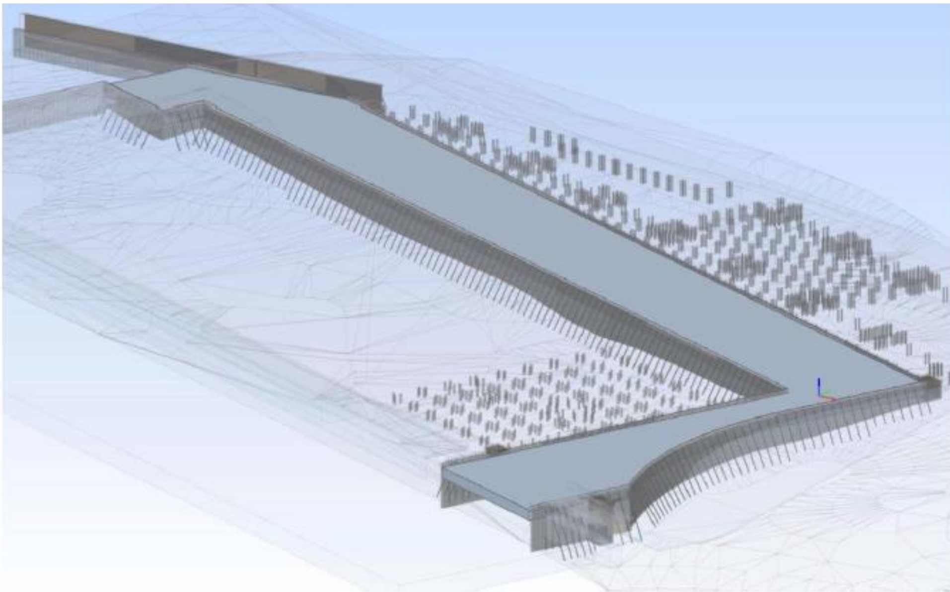
Modello BIM Canale e canaletto
