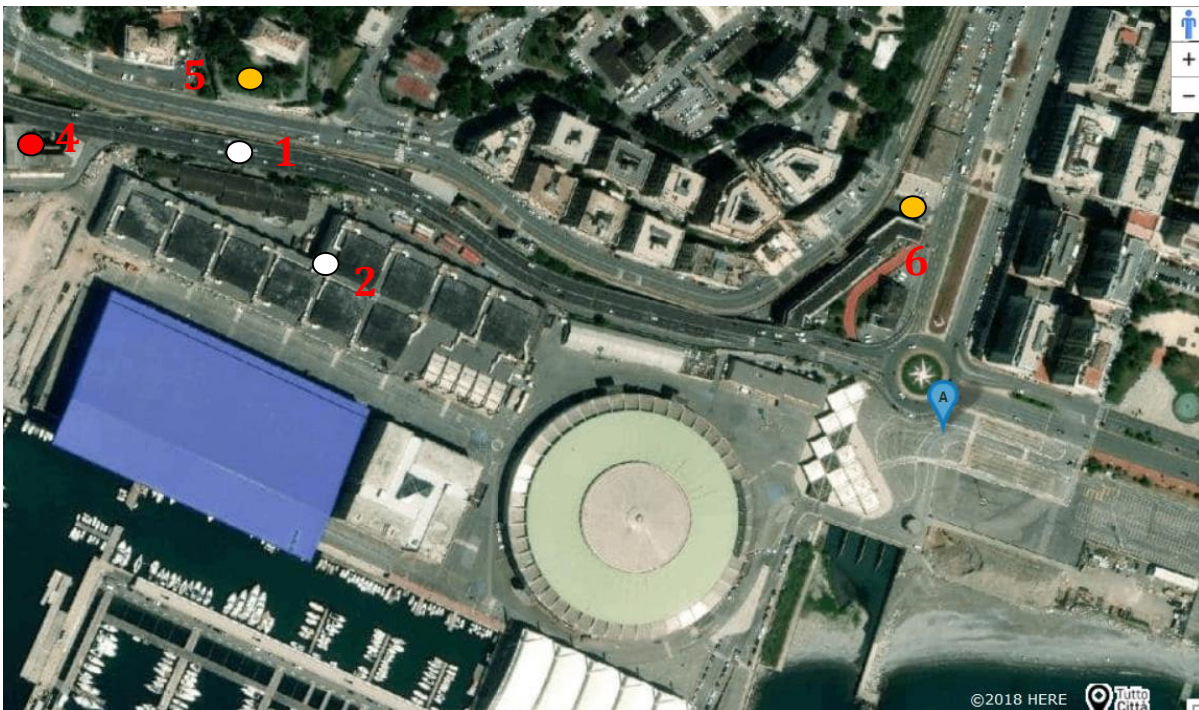
Mappa area di interesse con proposta di piazzamento stazioni di monitoraggio per demolizione padiglione M
